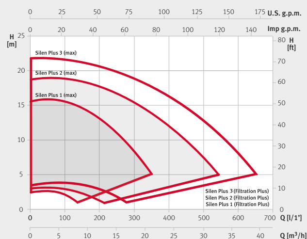
Curvas de funcionamiento
