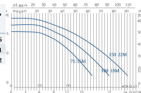
Curvas de funcionamiento a 2900 rpm
