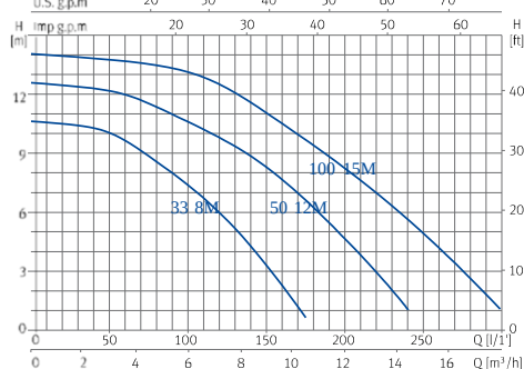
Curvas de funcionamiento a 2900 rpm
