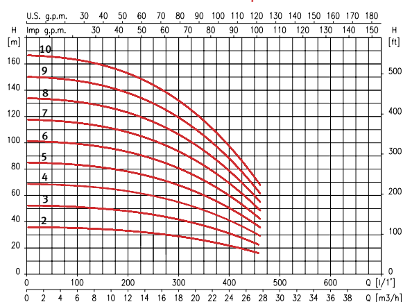
Curvas de funcionamento a 2900 rpm
