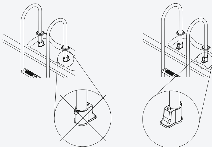
Fig. 1 - Colocação correta da tomada de terra.
