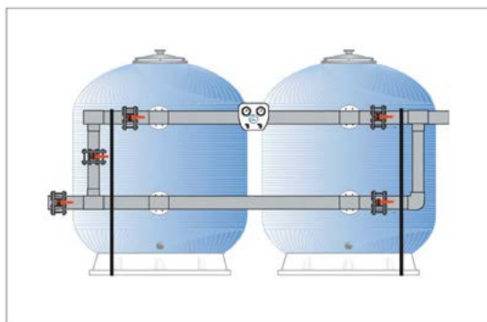
Esquema de instalação dupla
