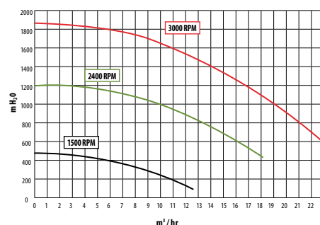
CURVAS DE RENDIMENTO / BOMBA RS II® VSTD 2,0 CV
