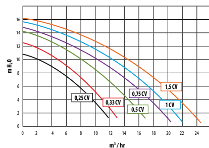
CURVAS DE RENDIMENTO / BOMBA POWERLINE PL
