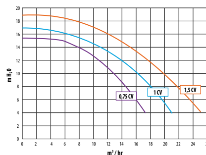
CURVAS DE RENDIMENTO / BOMBA ES TAGUS
