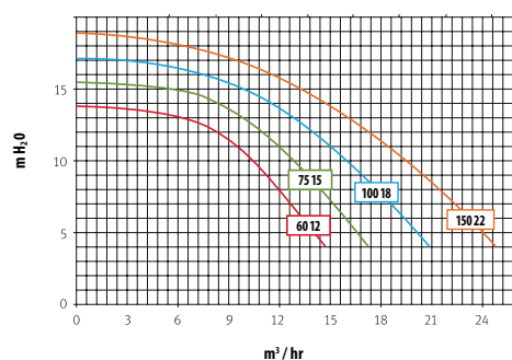
CURVAS DE RENDIMENTO / BOMBA SILEN S
