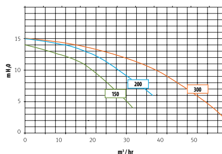
CURVAS DE RENDIMENTO / BOMBA WIPER 0 / 3
