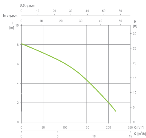
CURVAS DE RENDIMENTO / BOMBA KONA V 750M P A 2900 RPM
