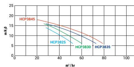
CURVAS DE RENDIMENTO / BOMBA HCP3800
