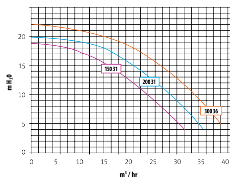
CURVAS DE RENDIMENTO / BOMBA SILEN S2
