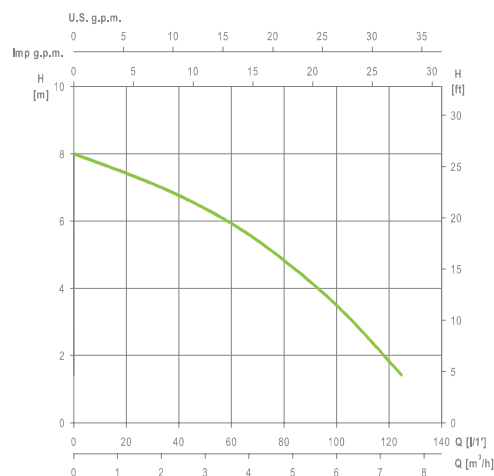
CURVAS DE RENDIMENTO / BOMBA KONA 400P M A 2900 RPM
