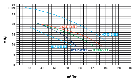
CURVAS DE RENDIMENTO / BOMBA HCP4000
