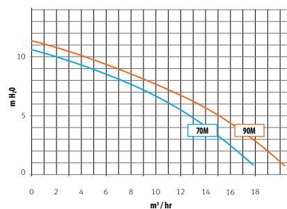
CURVAS DE RENDIMENTO / BOMBA TIPER
