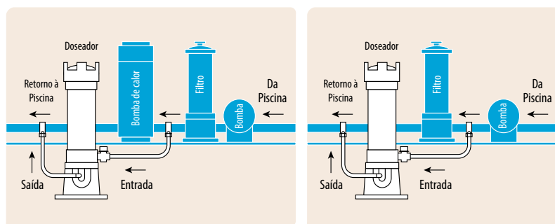
instalação off-line com bomba de calor
