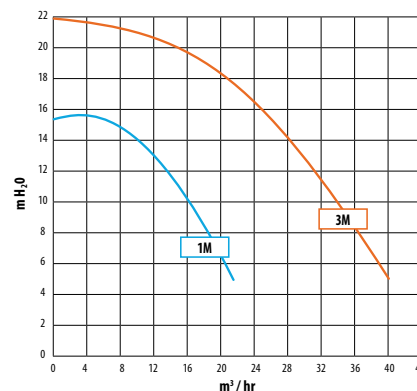
CURVAS DE RENDIMENTO / BOMBA SILEN PLUS
