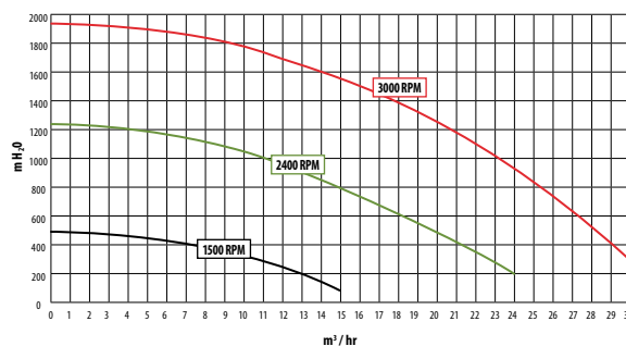
CURVAS DE RENDIMENTO / BOMBA RS II® VSTD 2,0 CV
