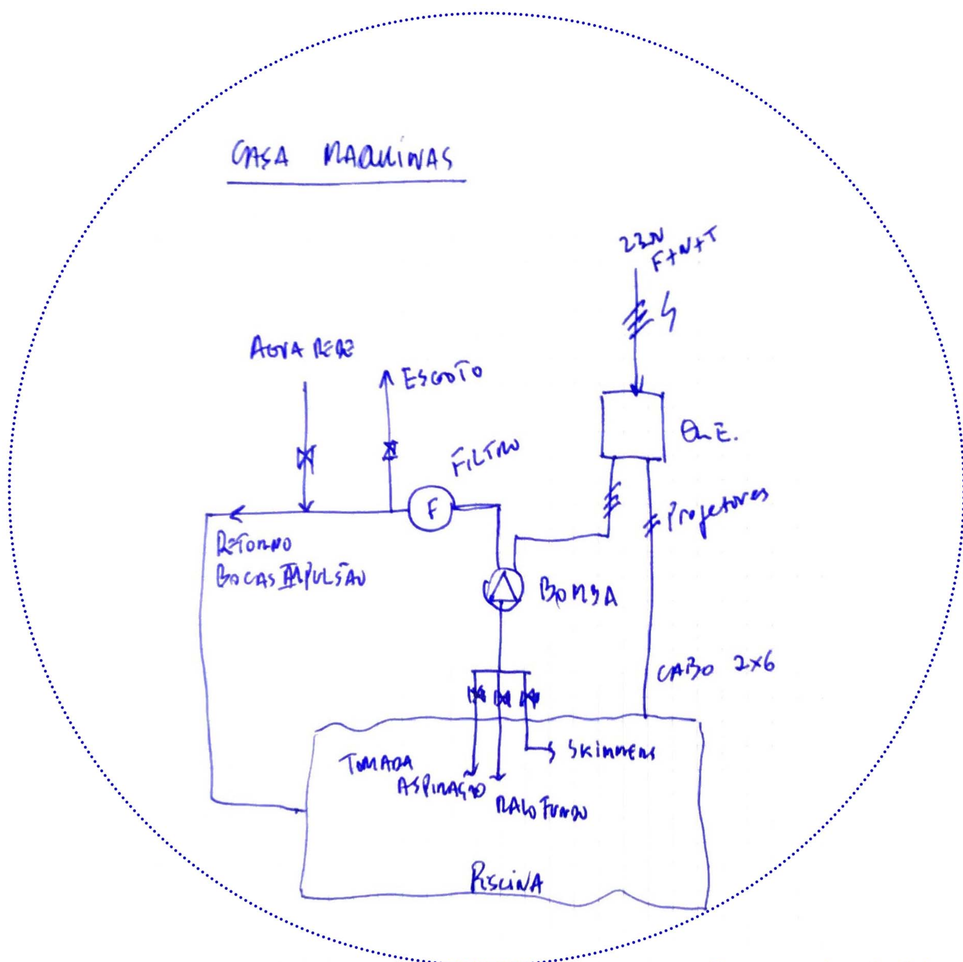
Esquema de princípio para piscina 9x4m
