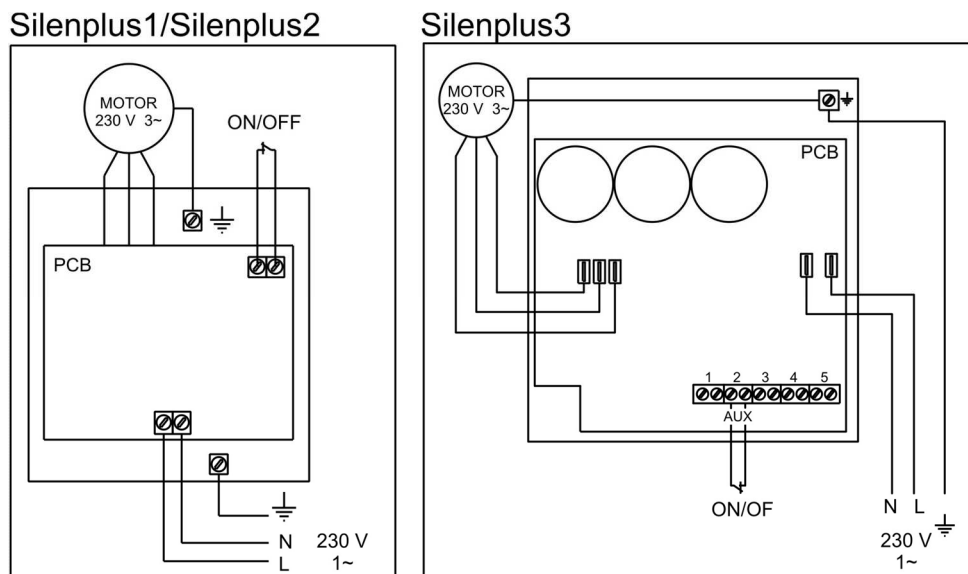
Esquema de conexiones / Connection Diagram / Schéma électrique / Schaltplan / Schema di collegamento / Aansluitschema
